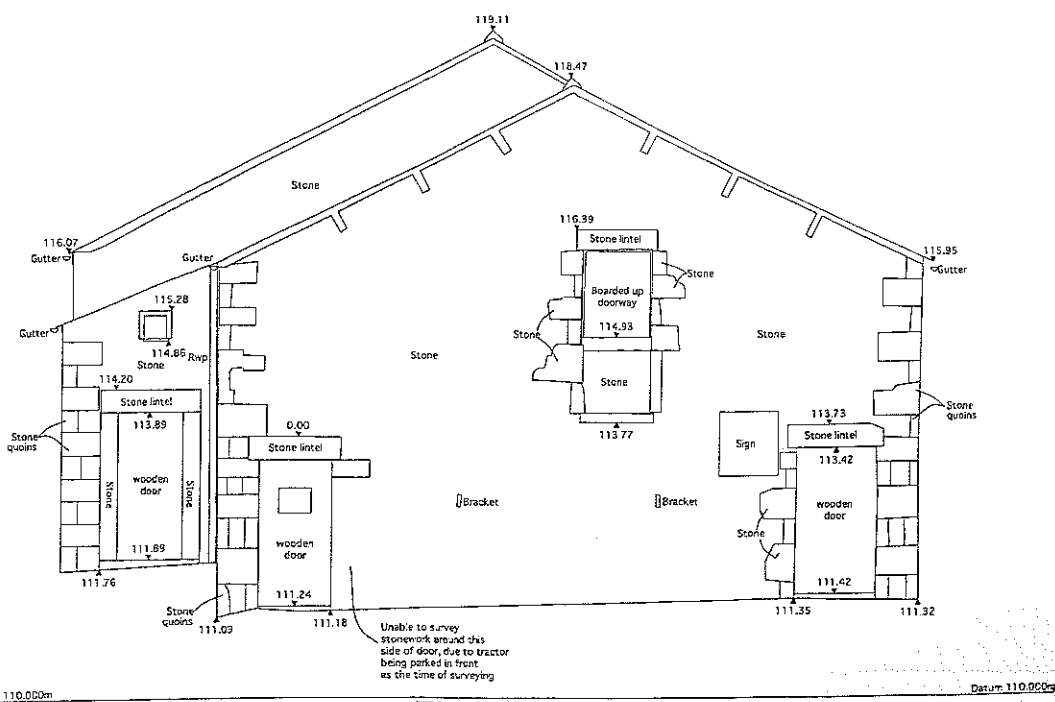
Elevation G
