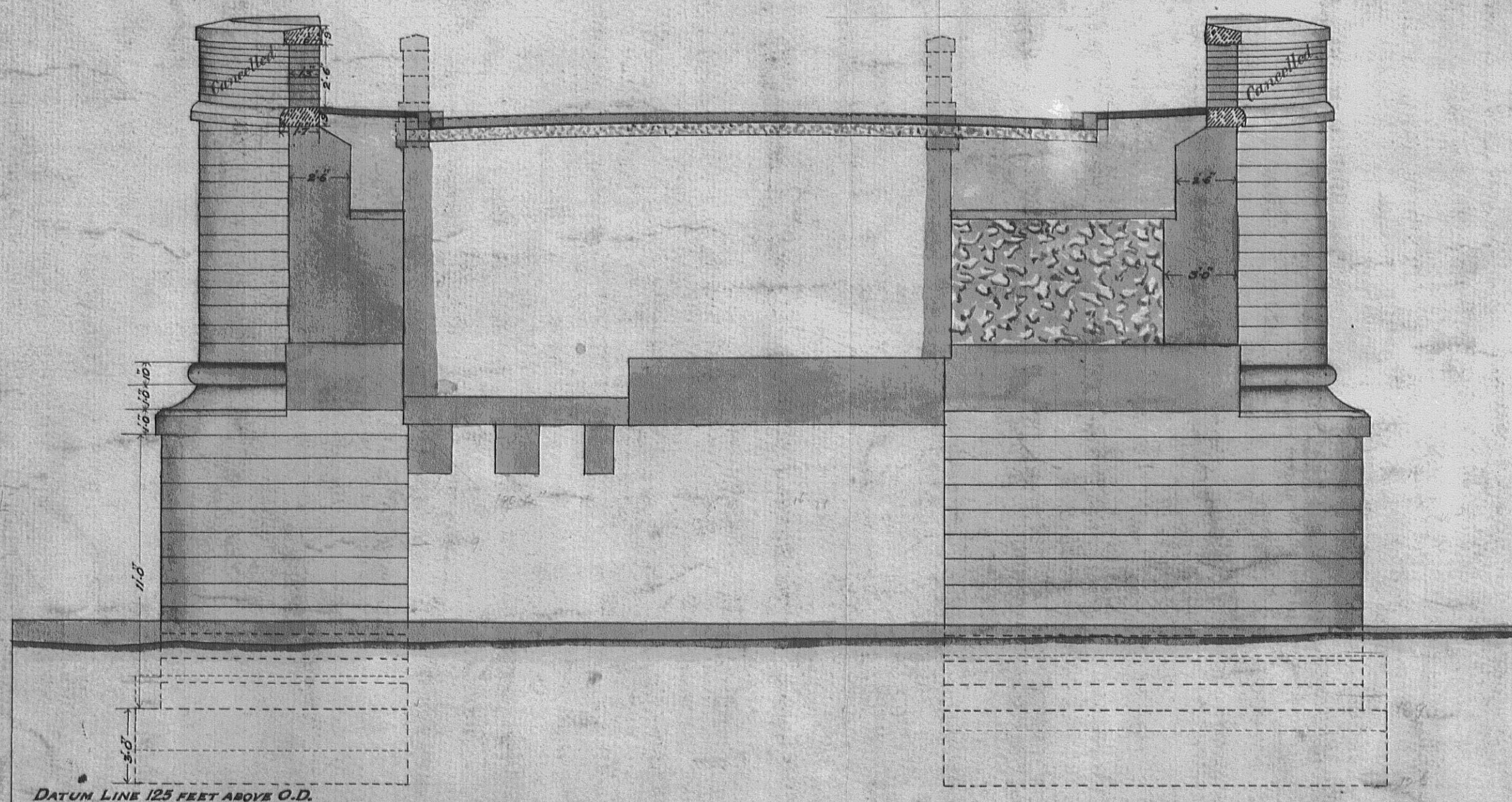
SECTION ON G.H.
