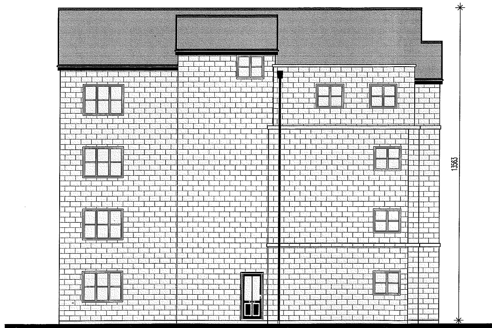
elevation 4
