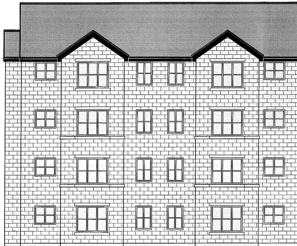
elevation 2
