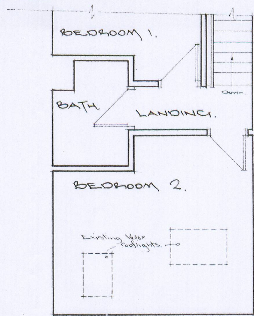
Existing F. F. plan. Scale: 1/4 to 60.
