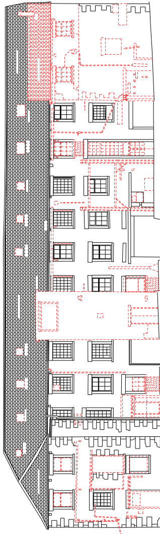
Elevation 01
