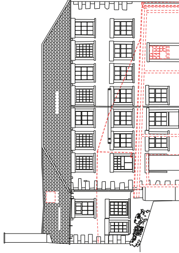
Elevation 02
