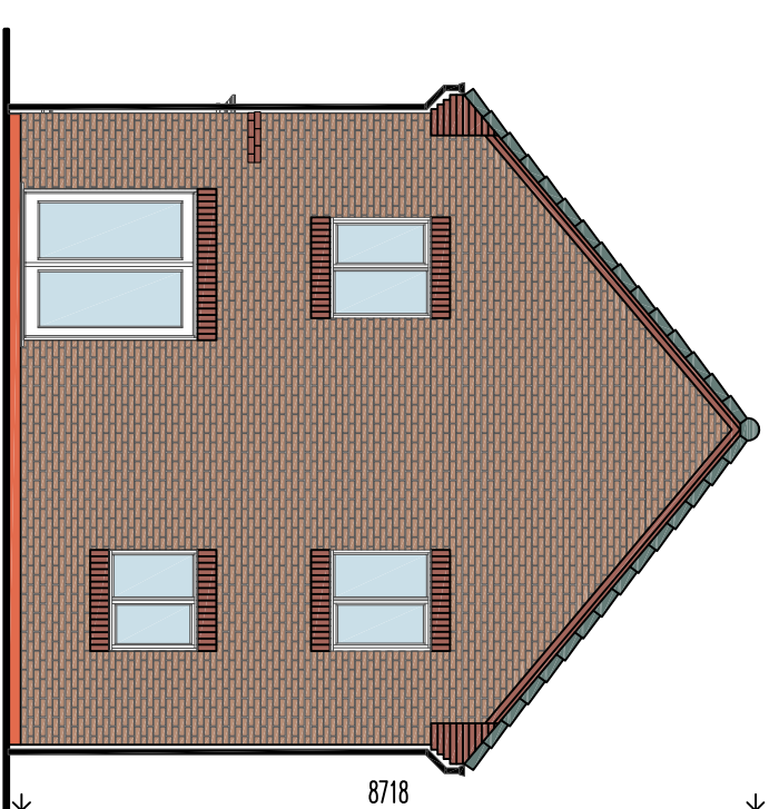
r.h. side elevation
