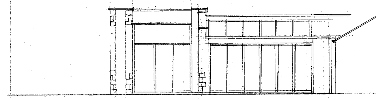
ELEVATION B
