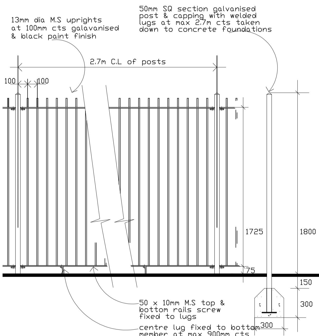
ELEVATION
