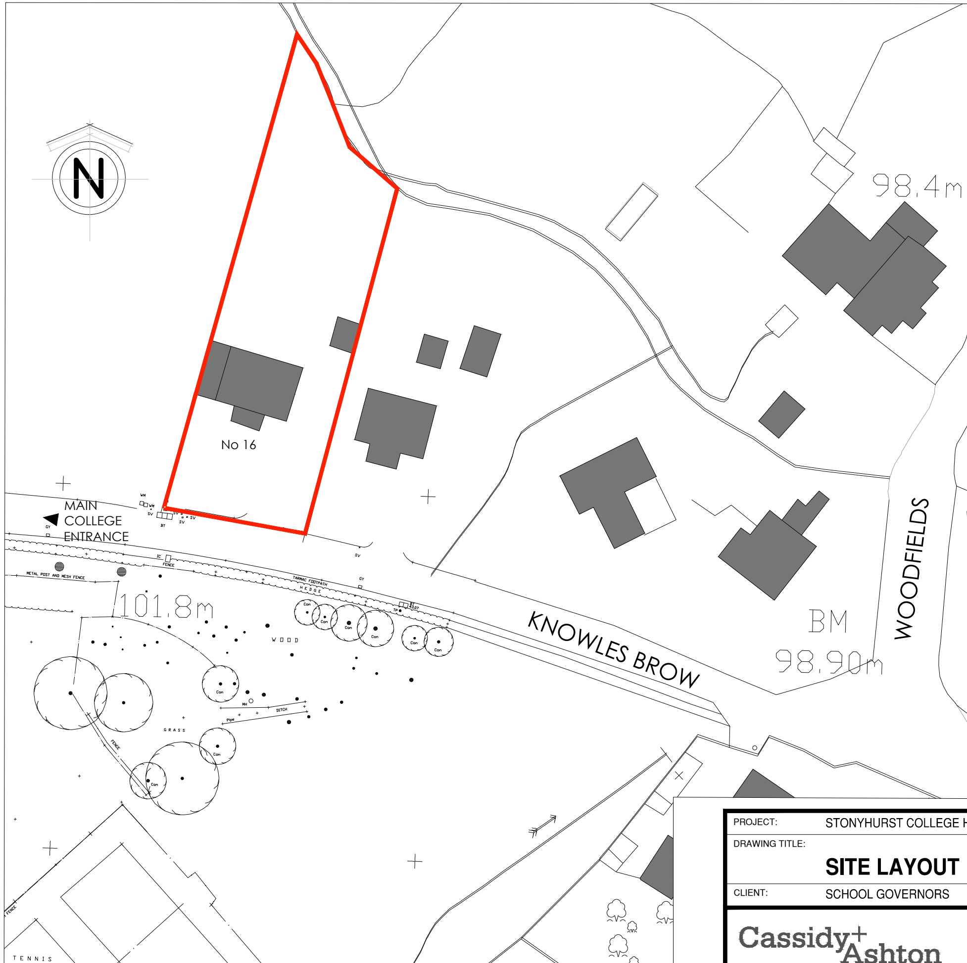
SITE PLAN 1:500
