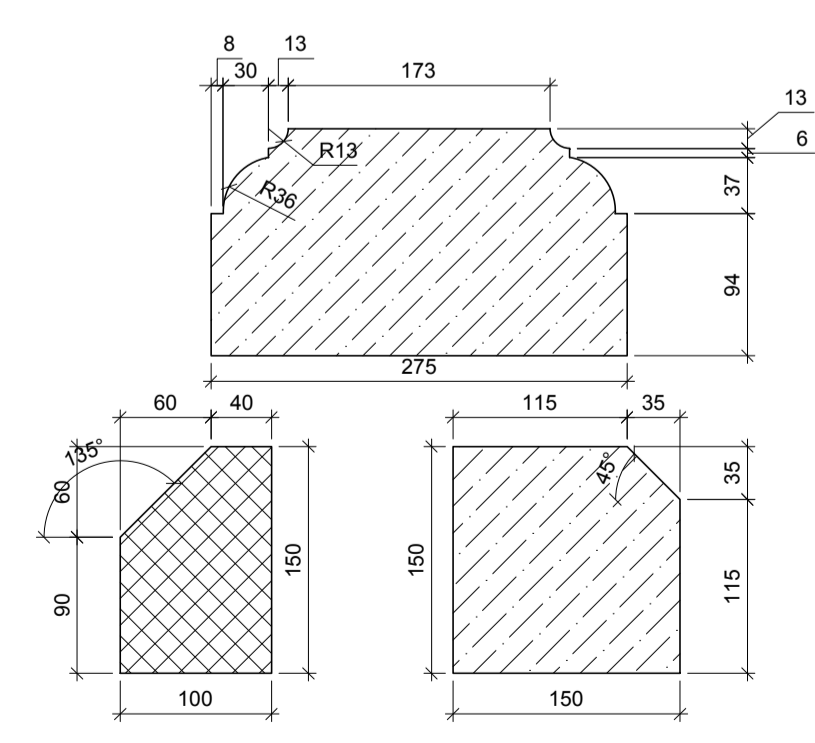
Plinth Detail 1:5
