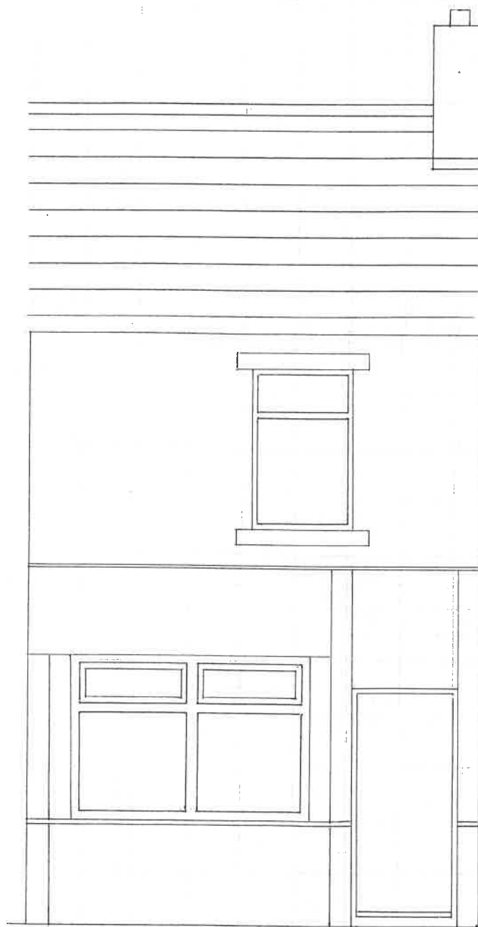
Existing 1:50
