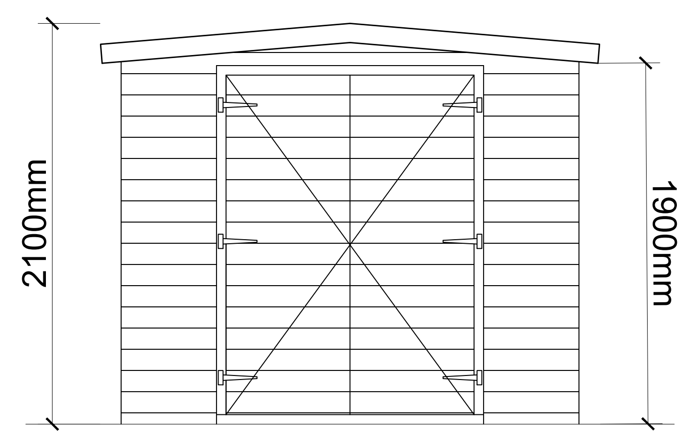
ELEVATION - A
