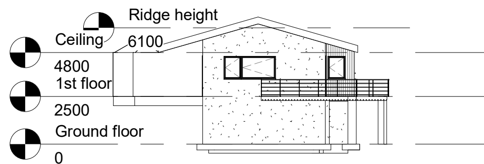
4 West 1 : 200
