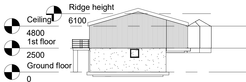
1 East 1 : 200
