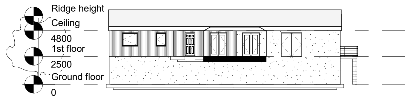
2 North 1 : 200
