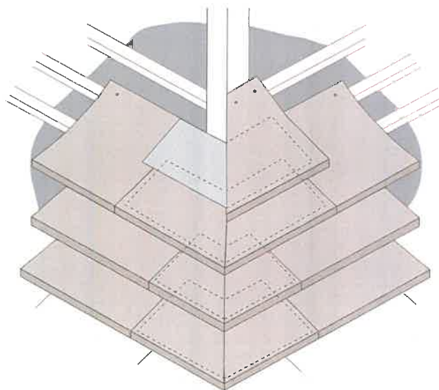
Mitred hip
