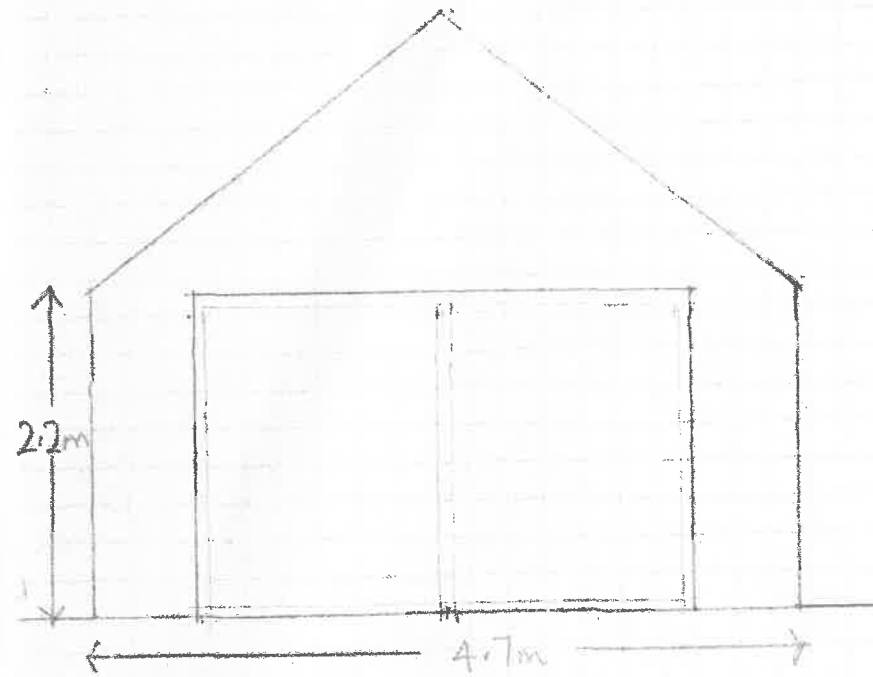
Elevation SE
