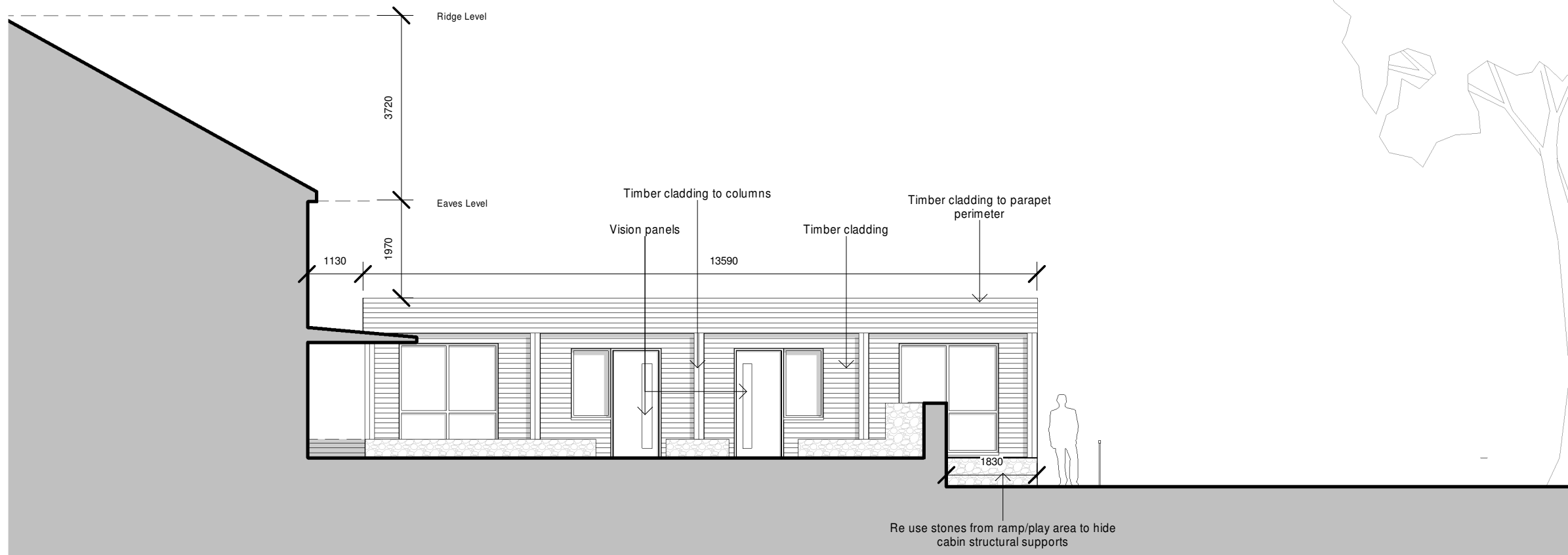
1 NW Elevation 1 : 100
