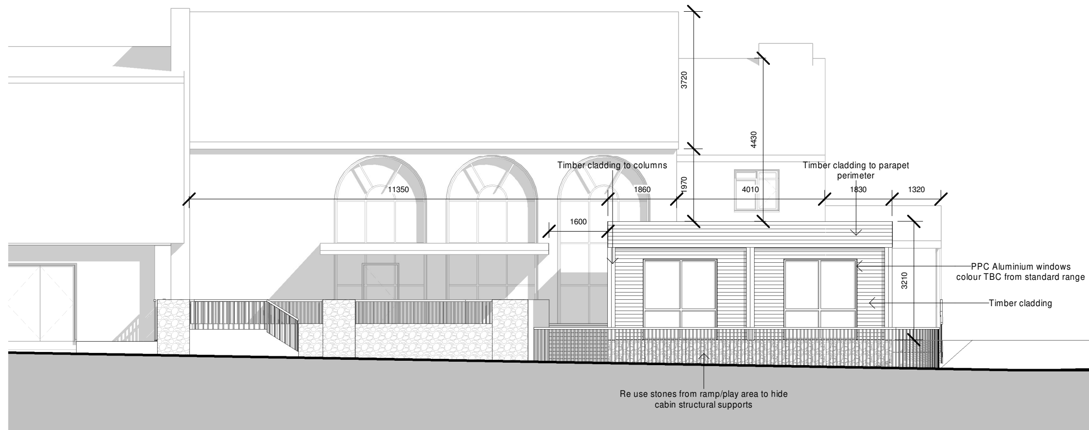
1 SW Elevation 1 : 100
