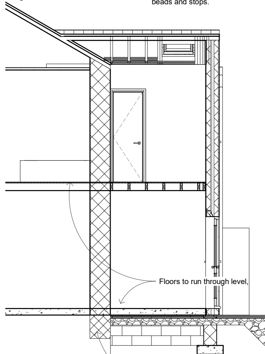
2 Section 3 1 : 50
