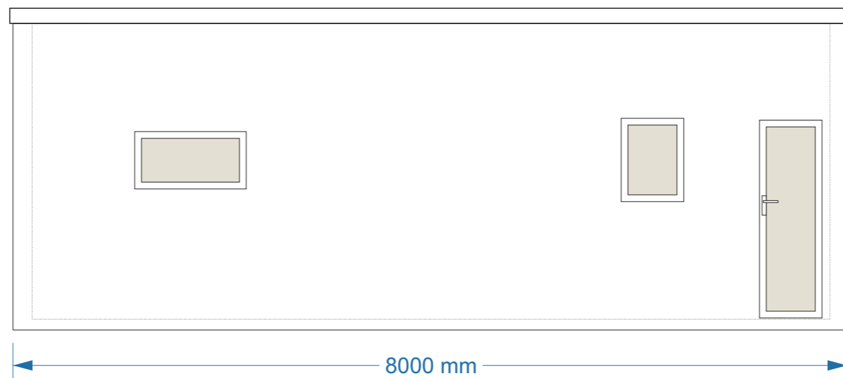
Right elevation
