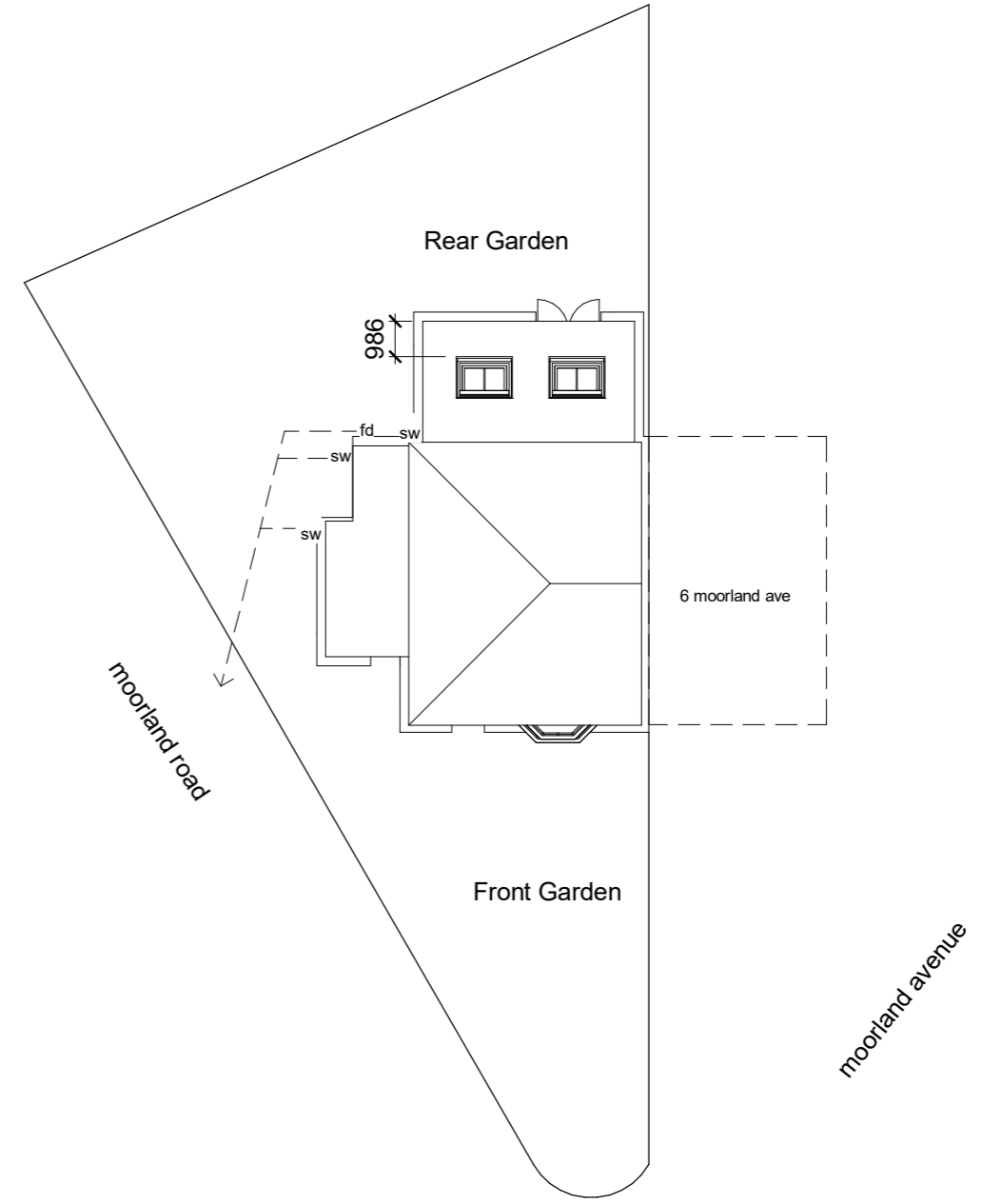
2 Site 1 : 200
