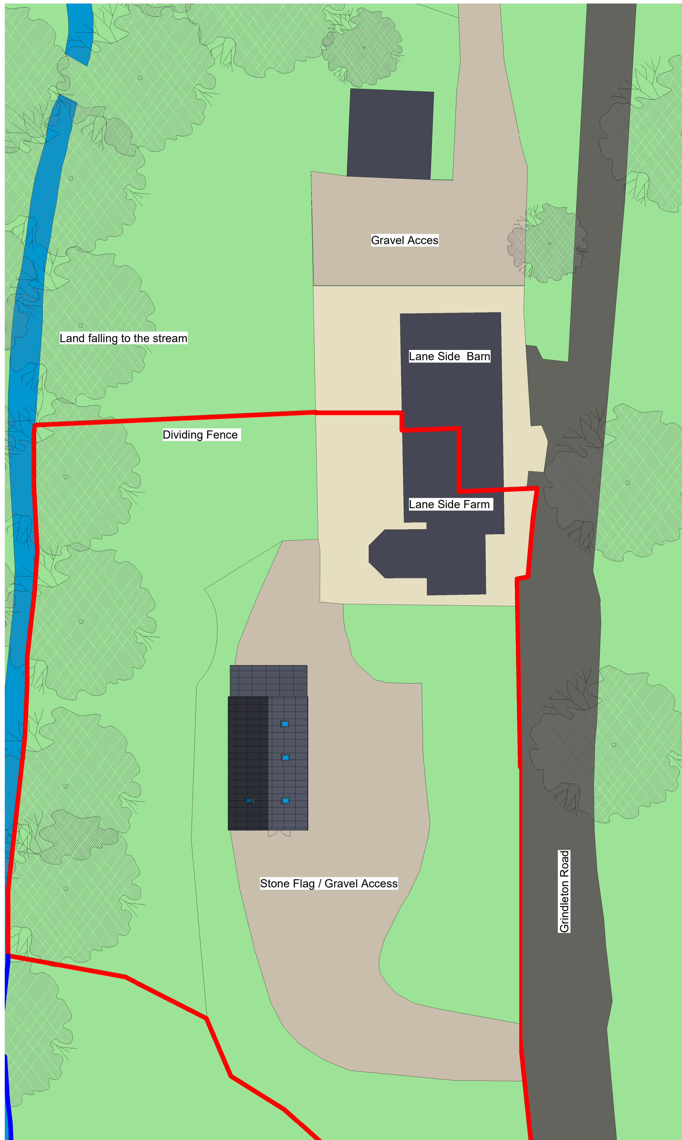
1 EXISTING SITE PLAN 1 : 200
