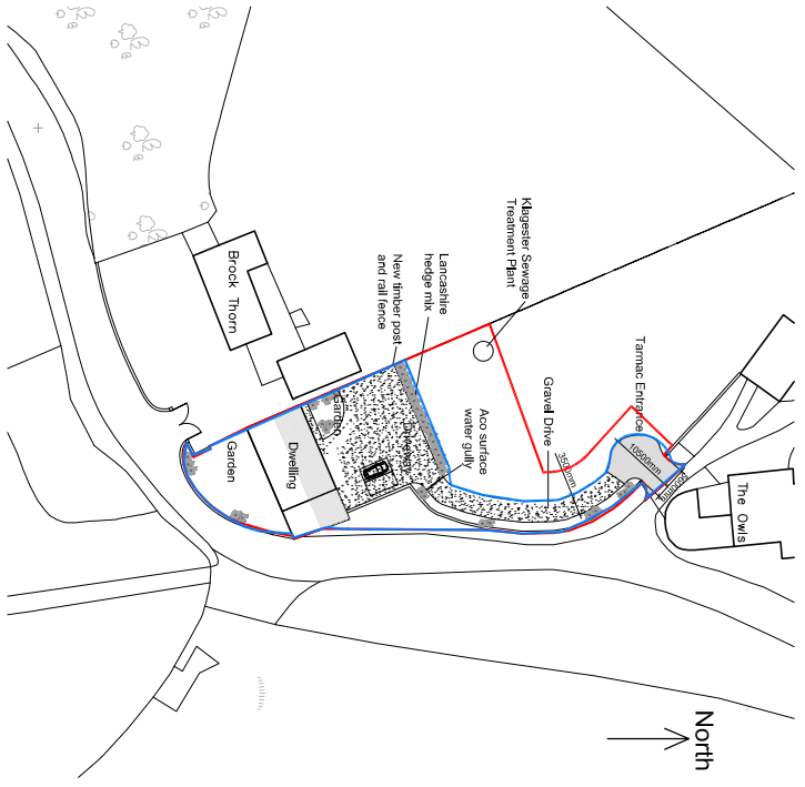
1:500 Site Plan
