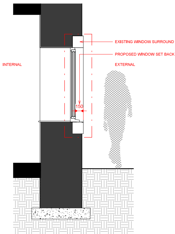
1 SECTION 1 : 20
