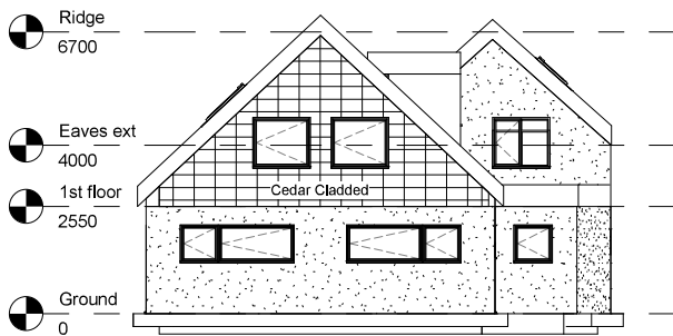
1 Front 1 : 100
