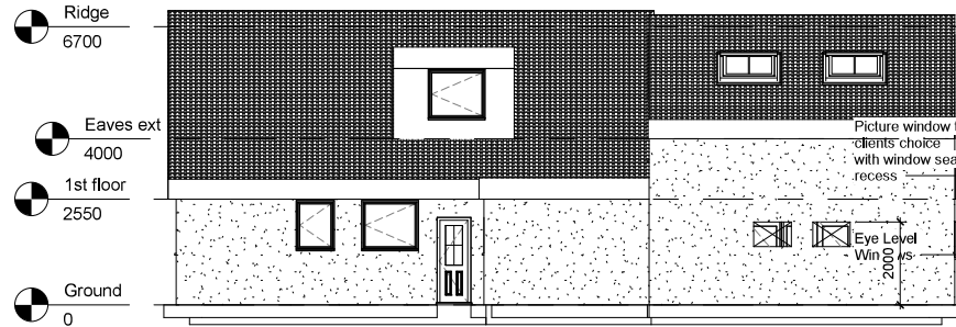
3 Side 1 : 100
