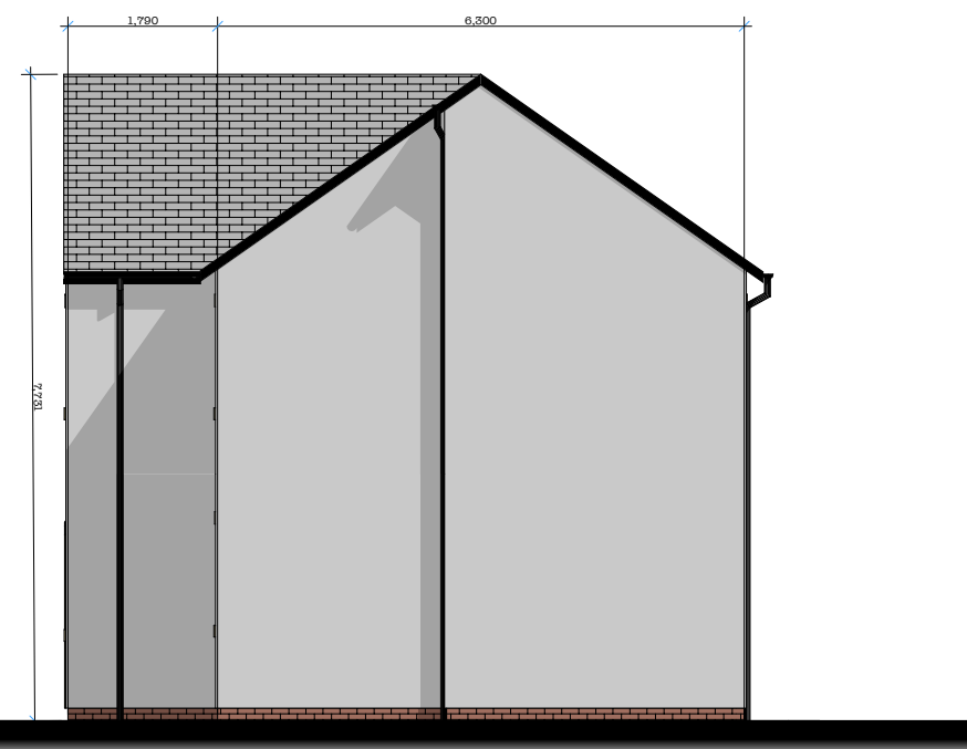
Side_2 elevation
