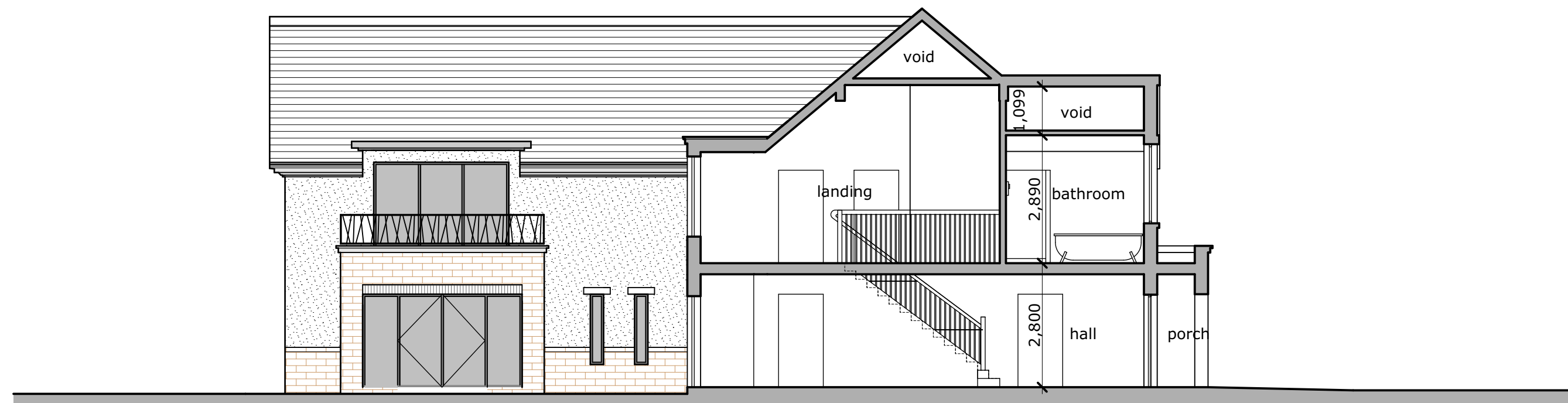
section A-A
