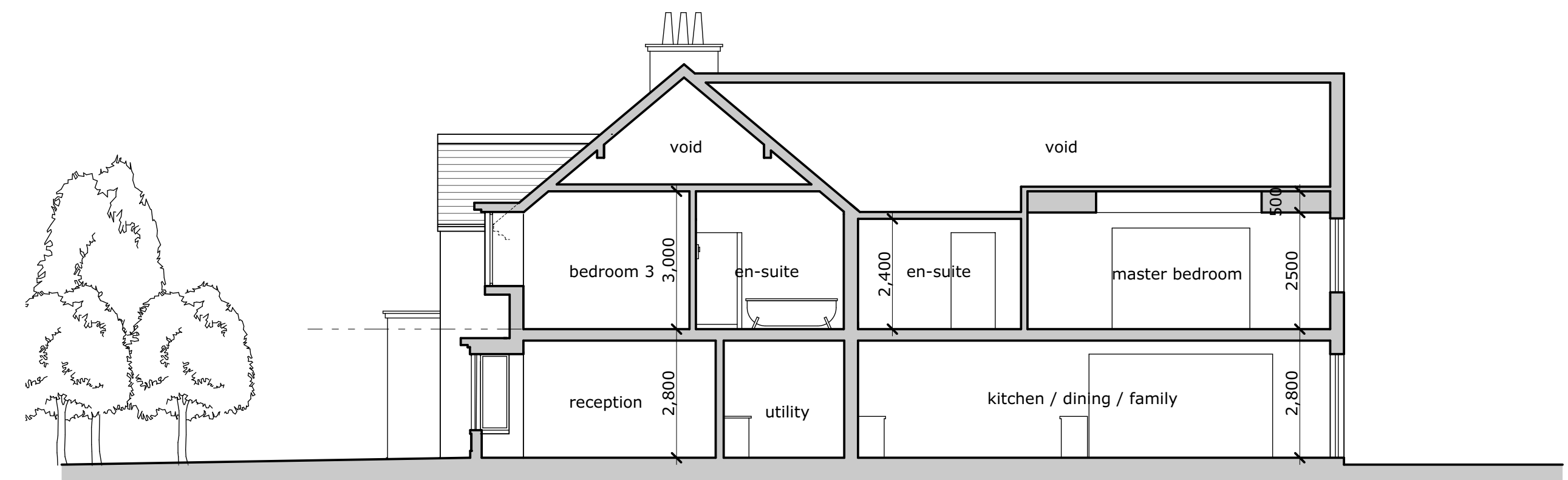
section D-D
