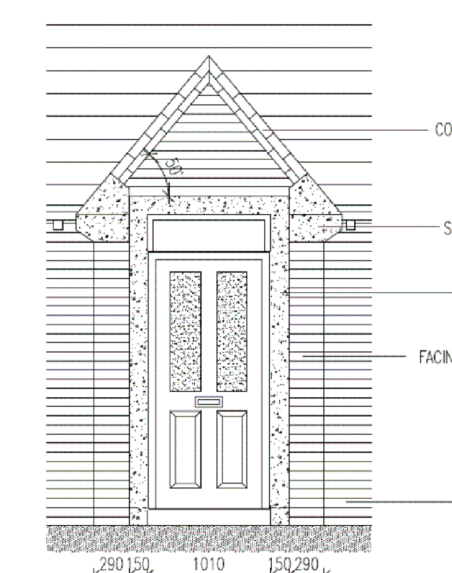
Porch detail (BUN3)
