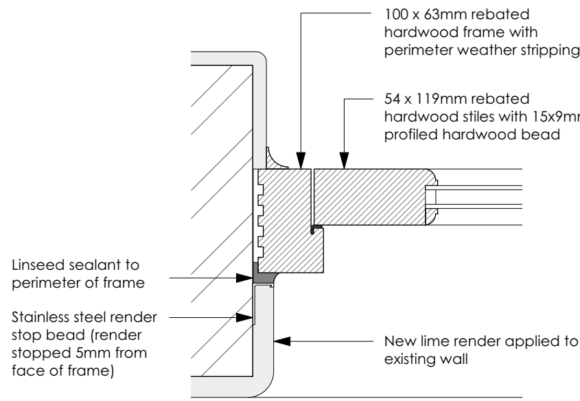
3 D.01 1:5
