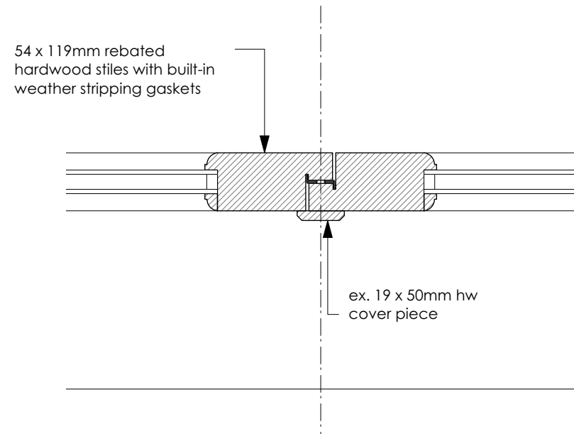
4 D.01 1:5
