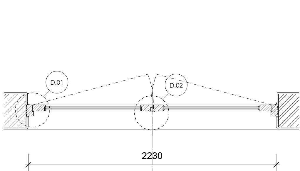
2 PLAN 1:20
