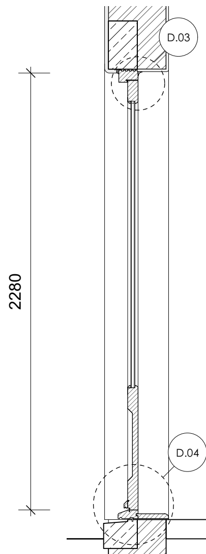
5 SECTION 1:20
