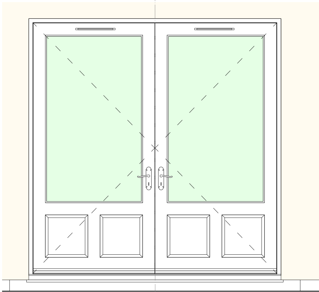
1 EXD.03 1:20
