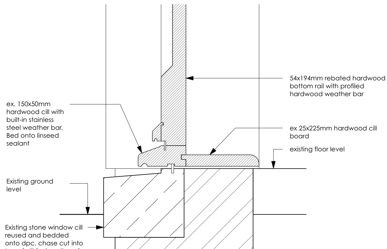
7 D.04 1:5
