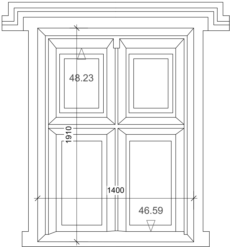
4 WG.01 1:20
