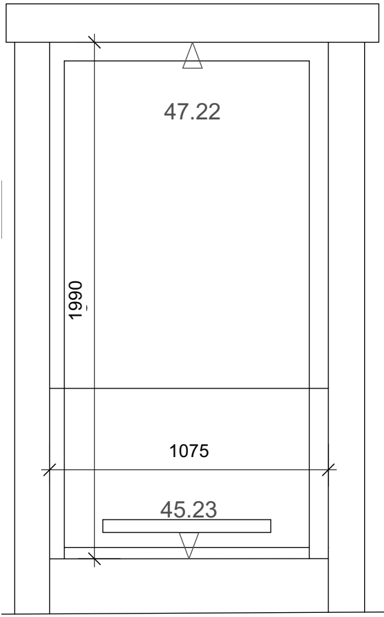
2 EXD.02 1:20
