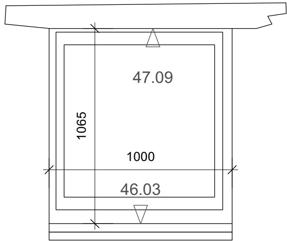
6 WG.03 1:20
