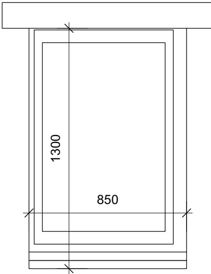
1 W1.01 1:20
