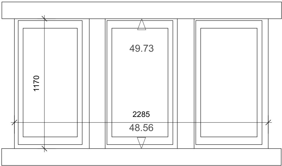
3 W1.03 1:20
