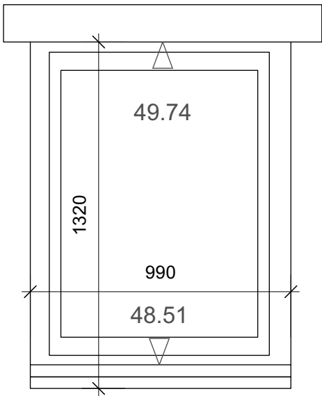
2 W1.02 1:20
