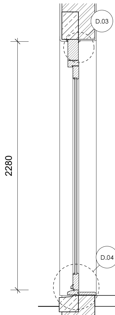
5 SECTION 1:20
