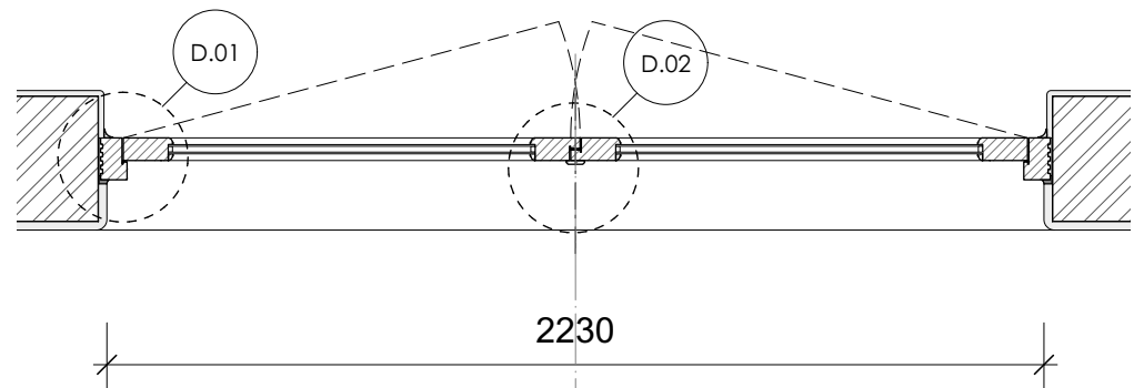
2 PLAN 1:20
