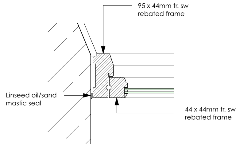
3 D.01 1:5
