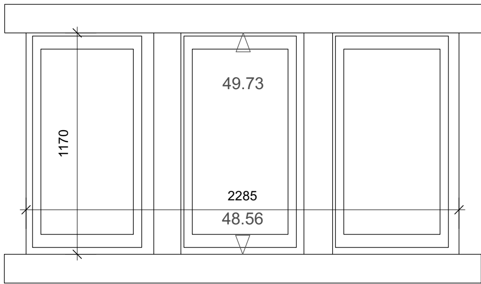
3 W1.03 + W1.04 1:20
