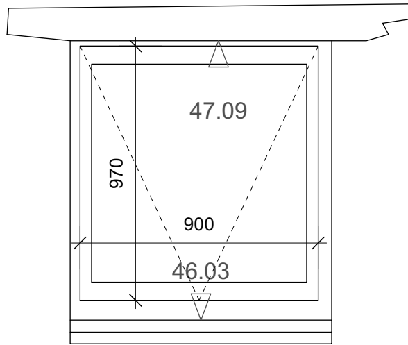
6 WG.03 1:20
