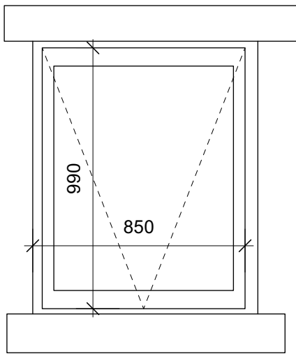
5 WG.02 1:20
