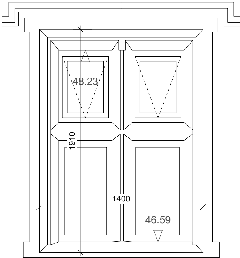
4 WG.01 1:20
