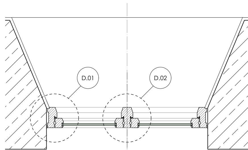
2 PLAN 1:10
