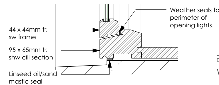
8 D.05 1:5
