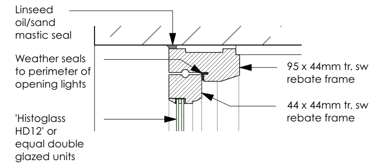
6 D.03 1:5
