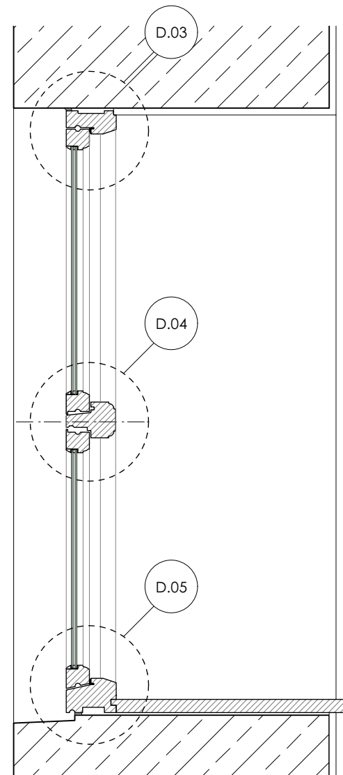
3 D.01 1:5
