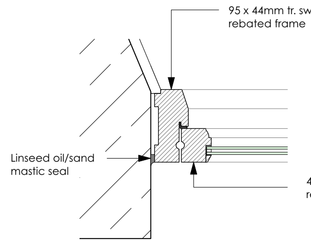
3 D.01 1:5
