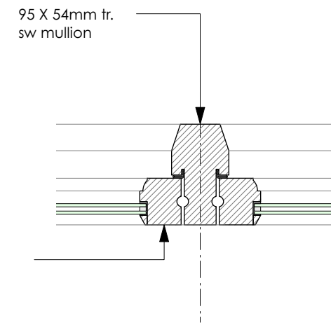
4 D.02 1:5
