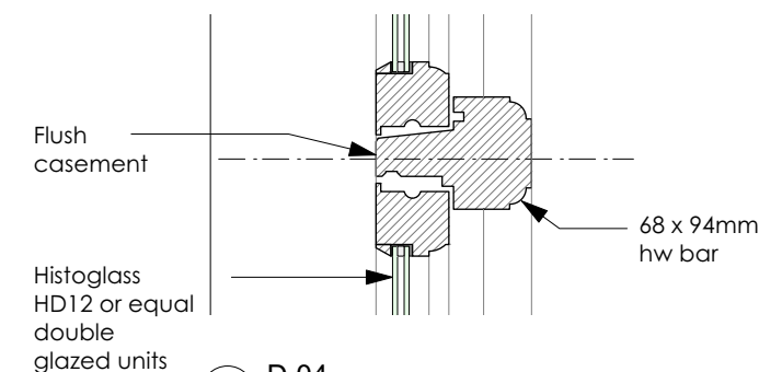
7 D.04 1:5
