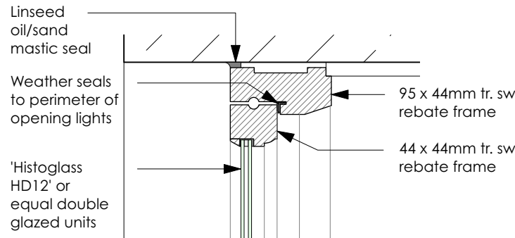
5 D.02 1:5
