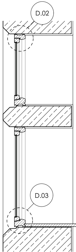
4 SECTION 1:20
