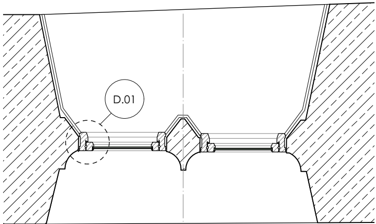
2 PLAN 1:20
