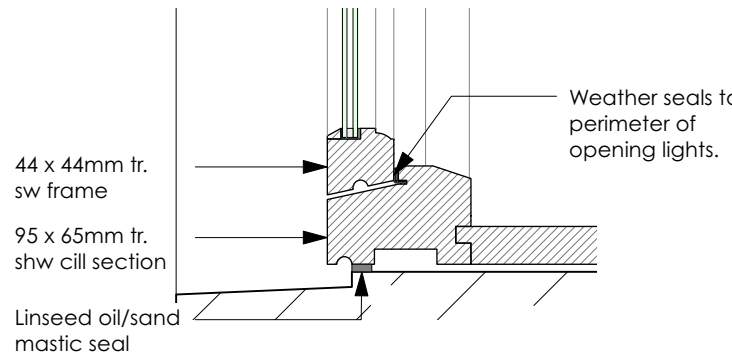
6 D.03 1:5
