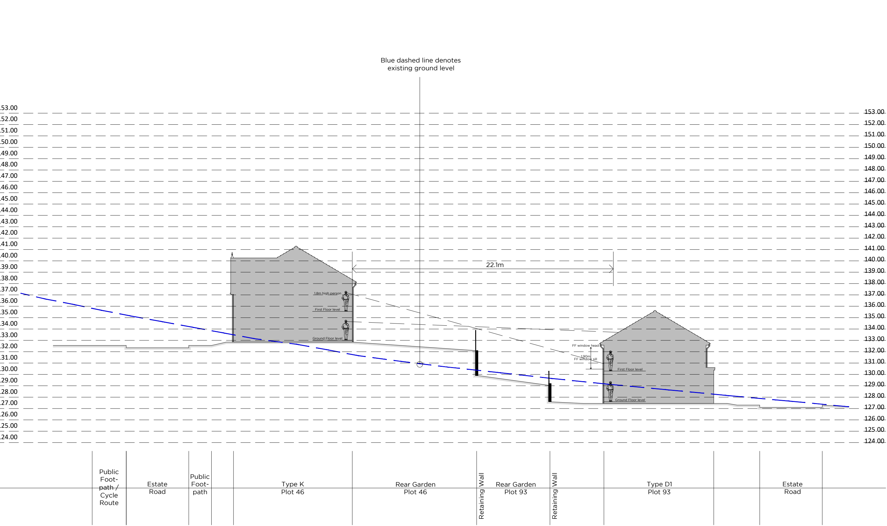
Site Section C - C
