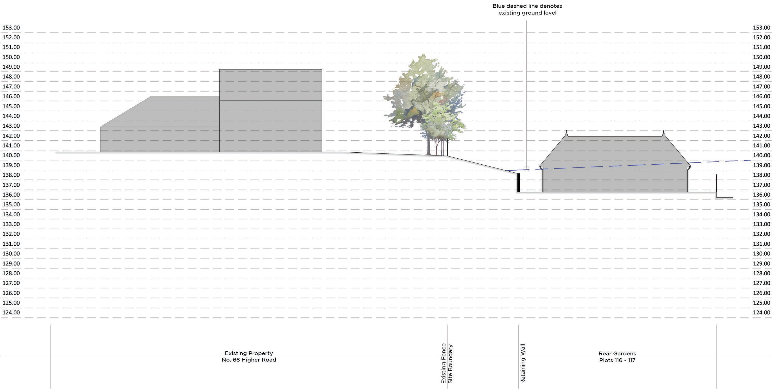
Site Section D - D
