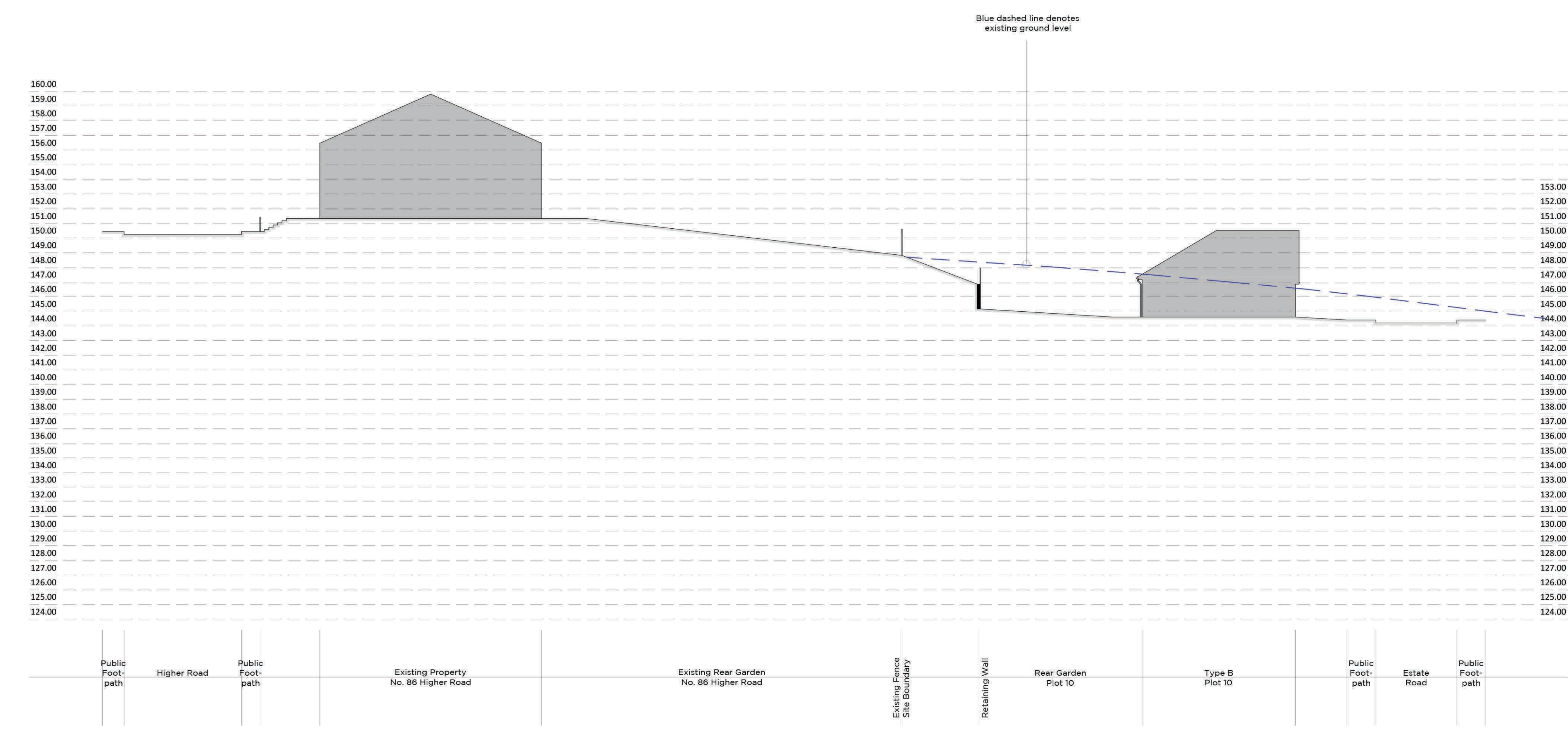
Site Section G - G
