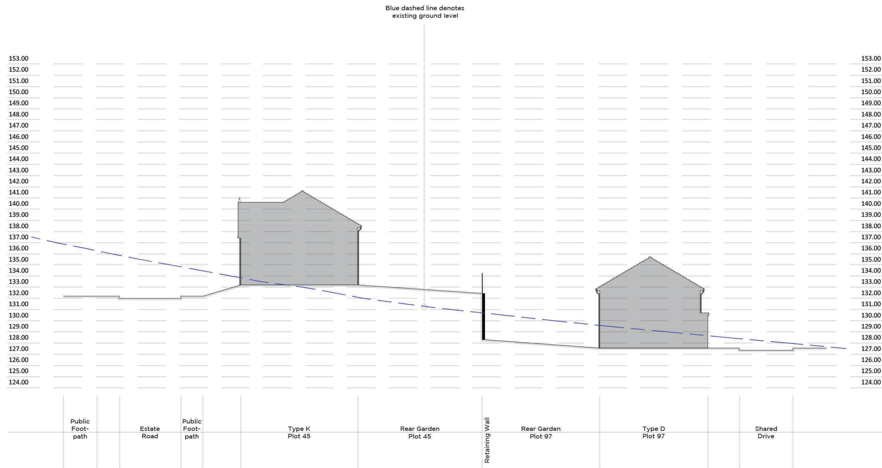
Site Section C - C
