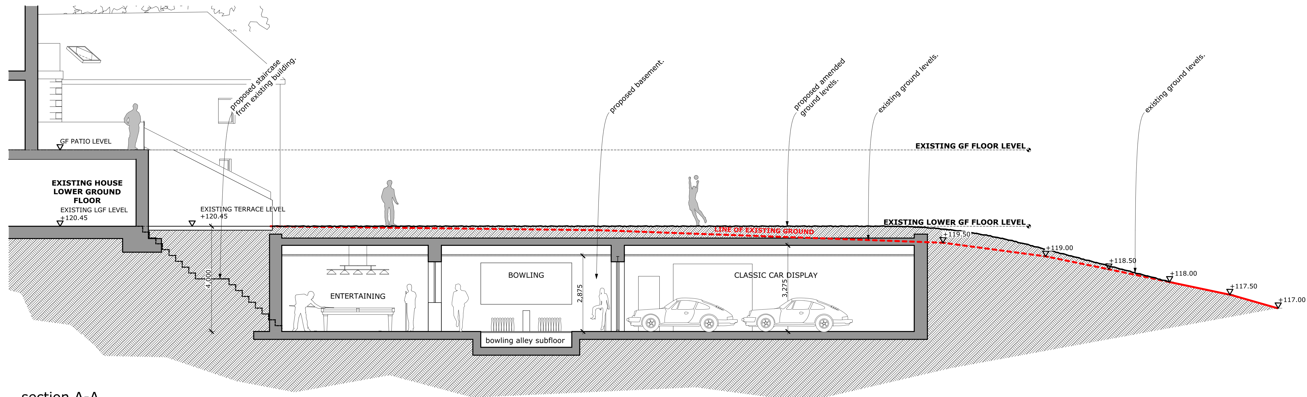
section A-A
