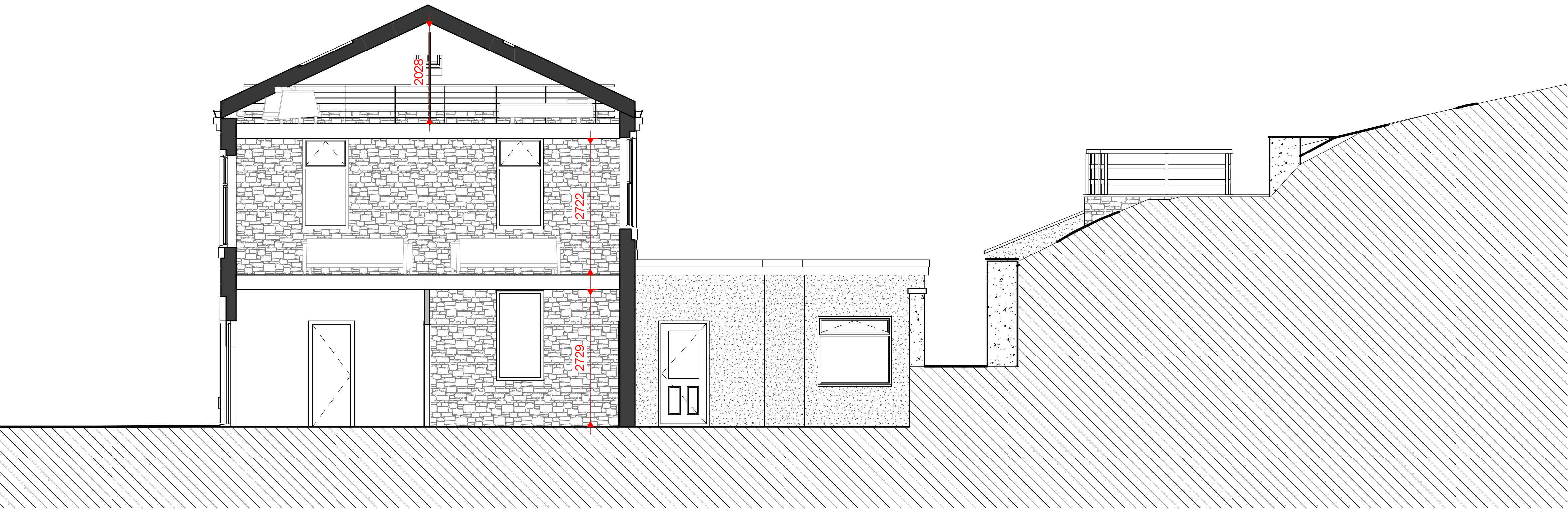
1 Section 3 1 : 50
