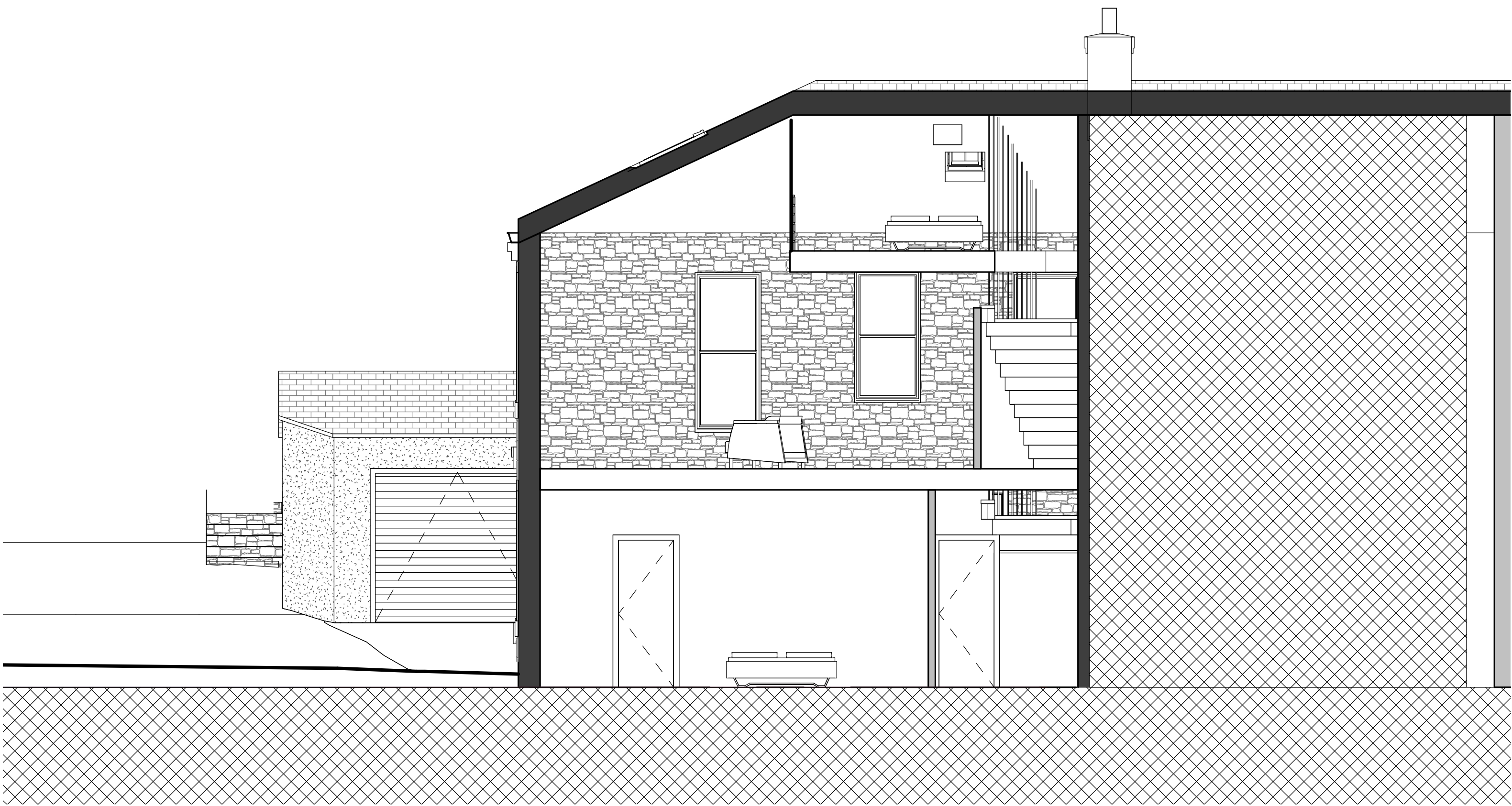
2 Section 5 1 : 50
