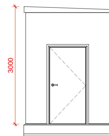
ELEVATION F 1 : 50
