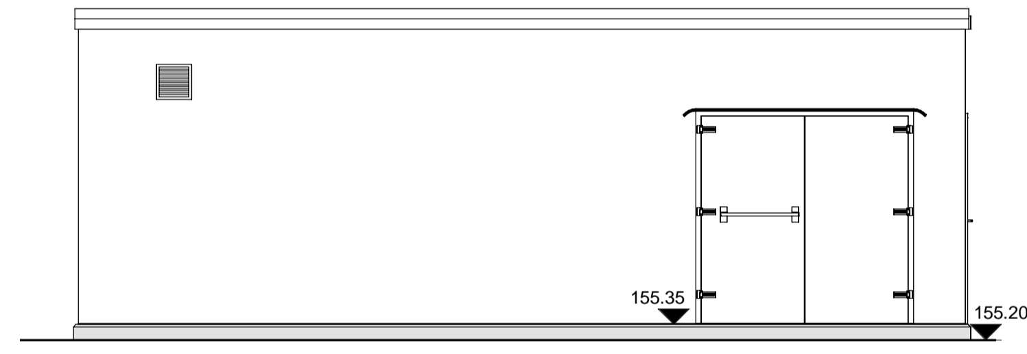
ELEVATION A 1 : 50
