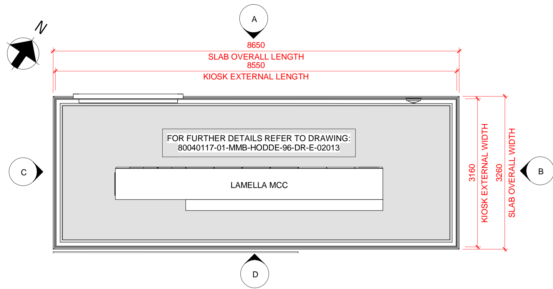
MCC KIOSK DETAILS 1 : 50
