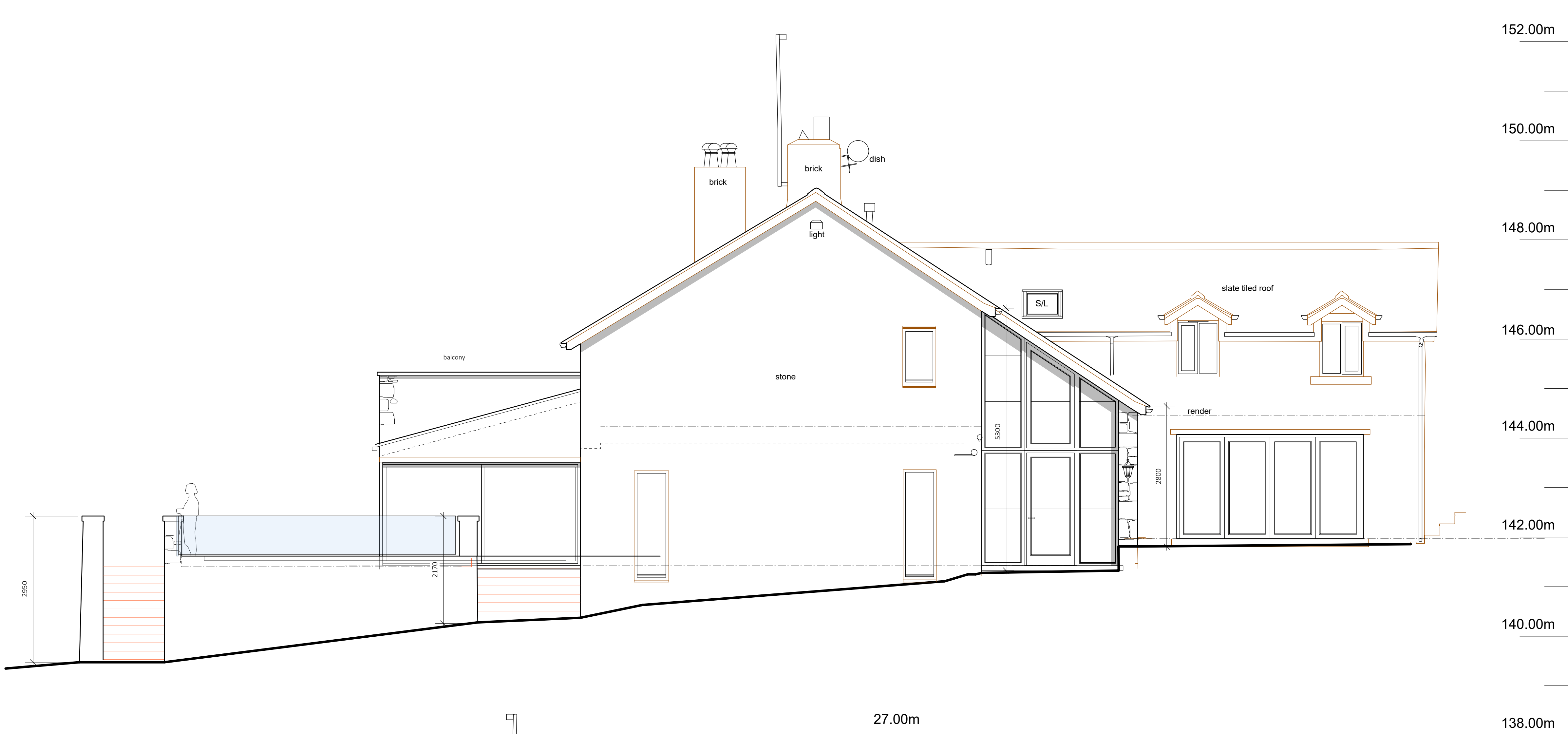
ELEVATION B-B
