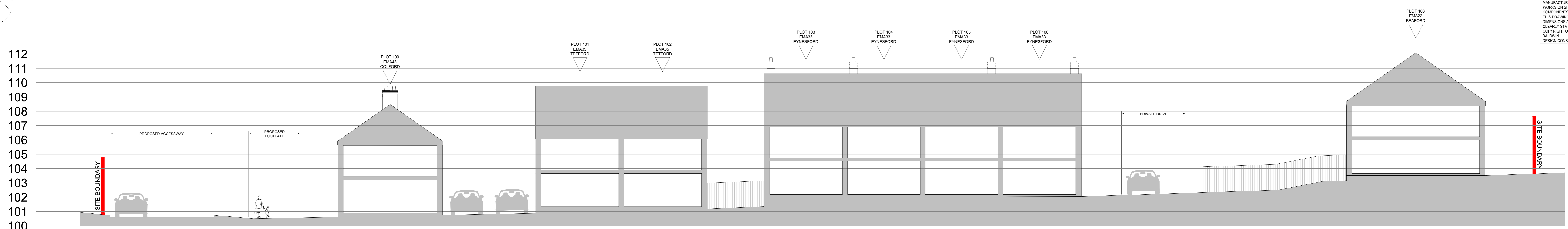
Site Section A-A
