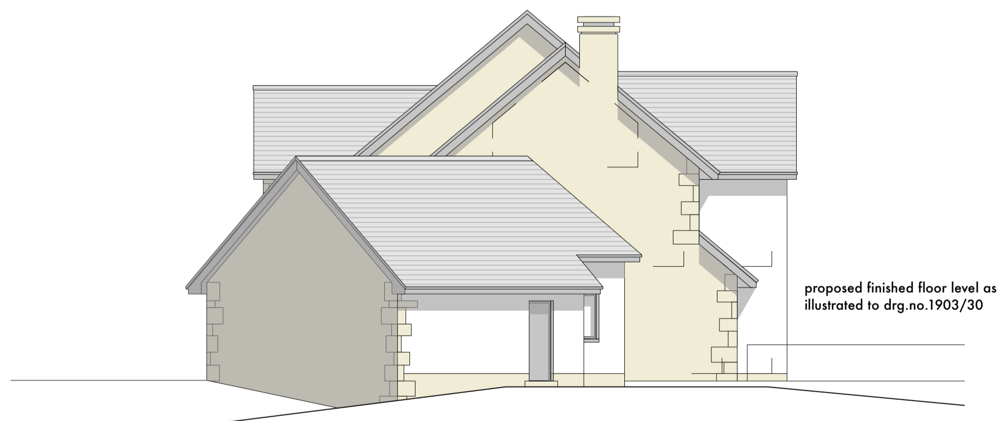
elevation 3
