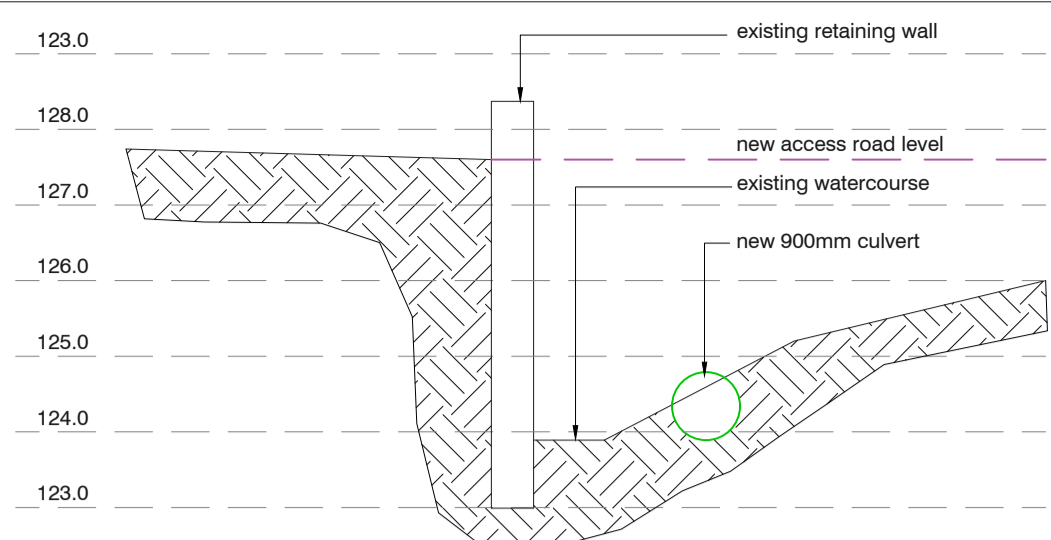
SECTION A-A 1:100 scale
