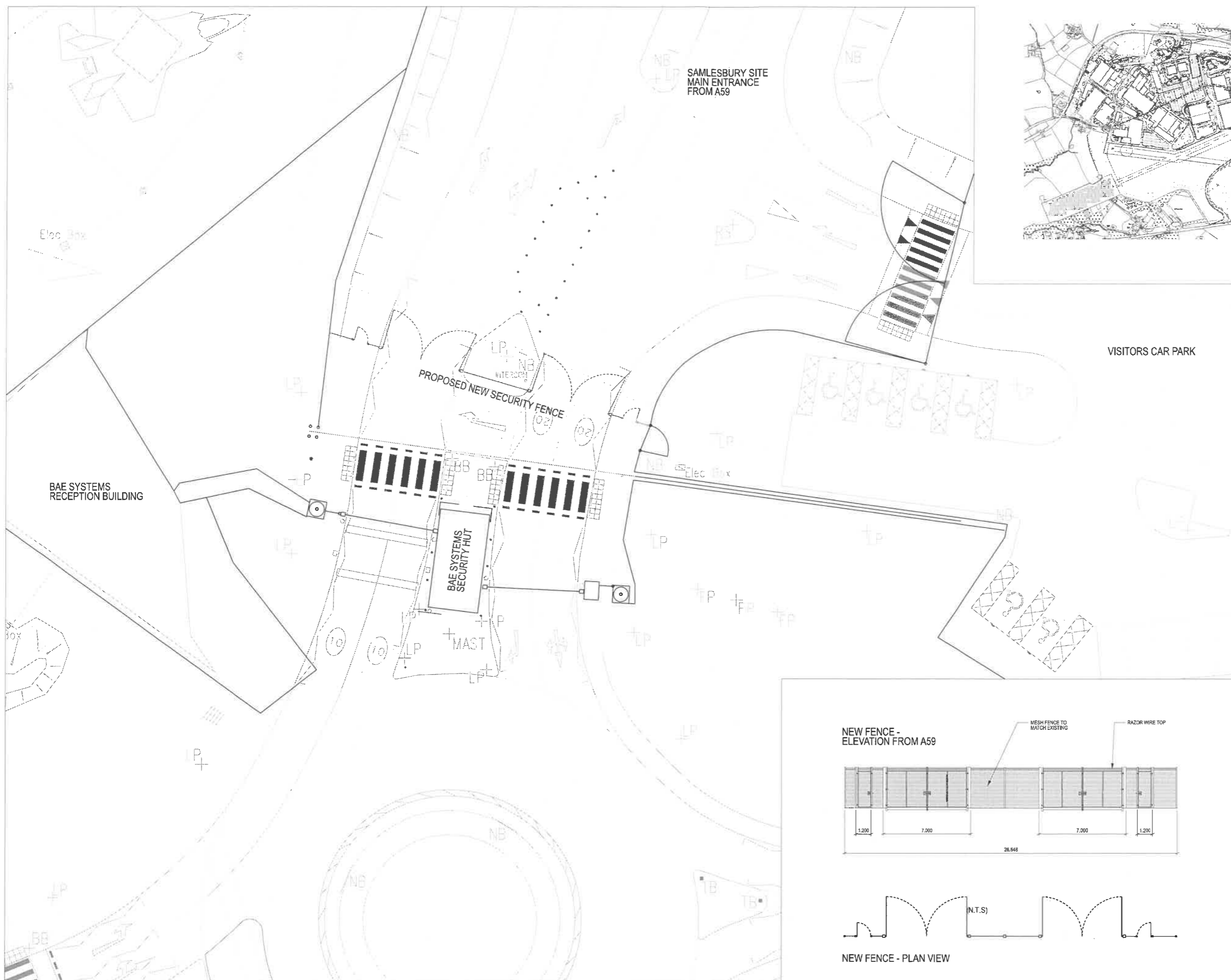
SAMLESBURY SITE LOCATION PLAN N.T.S.
