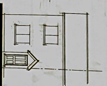
SE ELEV
