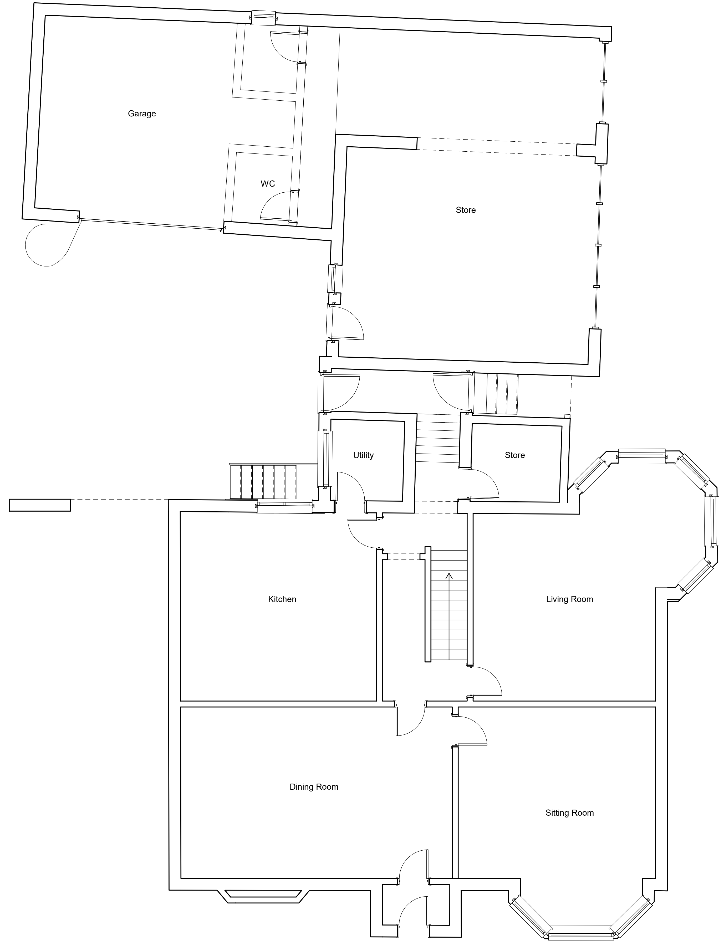
1 Extension Floor 1 : 50
